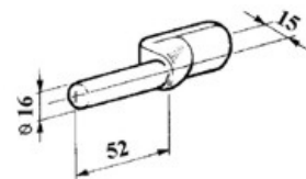
art. 20108 PERNO D. 16 BASSO gr. 200
