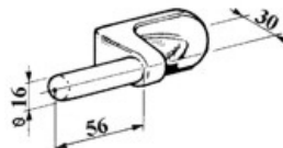
art. 20114 PERNO D. 16 ALTO gr. 230
