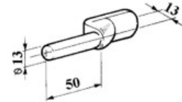
art. 20102 PERNO D. 13 gr. 110
