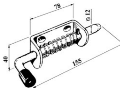
art. 20132 PERNO A MOLLA ZINCATO gr. 300
