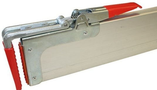
art. 31420 FERMA CARICO IN ALLUMINIO mm 1980/2700 Gr. 9.500
