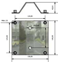
R8278004 F08-TL Piedino di supporto centrale in acciaio zincato con inseri filettati M8 Zinc plated steel foot mounting support with M8 threaded inserts
