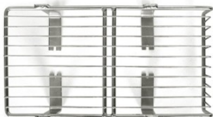
GRIGLIA PARASASSI Montaggio su BARRA
