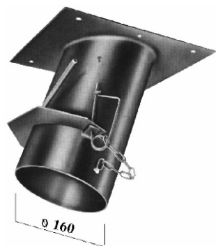
art. 55074 BOCCHETTA SCARICO CEREALI gr. 4.800
