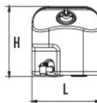
art. 55224 TANICA ACQUA IDRO 25 CON PORTASAPONE L 300 x P 495 x H 303 gr. 2.600 (lt. 25)
