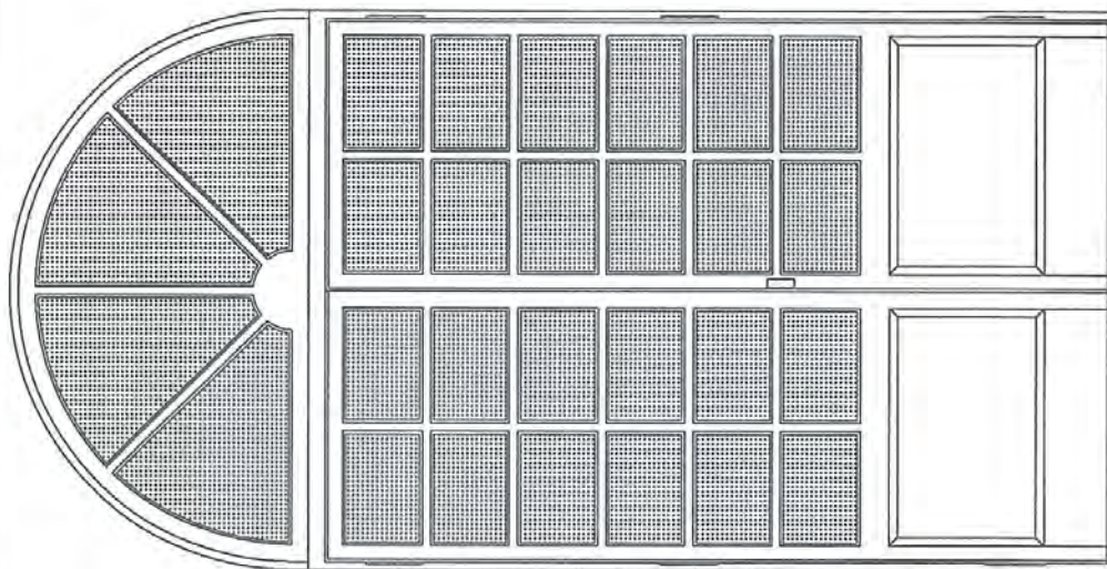
STATO di FATTO - Serramento porta tipo H
