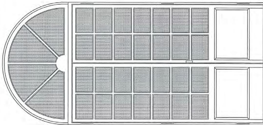
PROGETTO - Serramento porta tipo H
