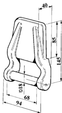
art. 15236 CERNIERA PESANTE gr. 1.250
