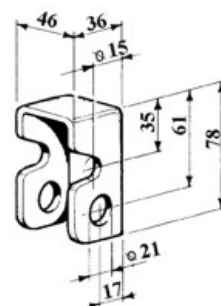
art. 15350 SUPPORTO GUIDA ASTA gr. 250
