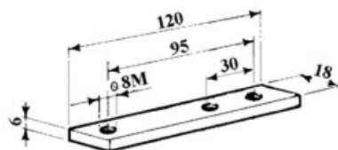
art. 15285 PIASTRINA gr. 95
