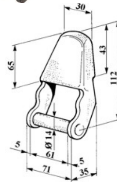
art. 15206 CERNIERA T/PARIPIANALE gr. 340
