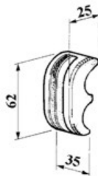
art. 15214 PALETTA gr. 140
