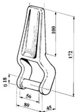
art. 15216 CERNIERA PESANTE ALTA gr. 920
