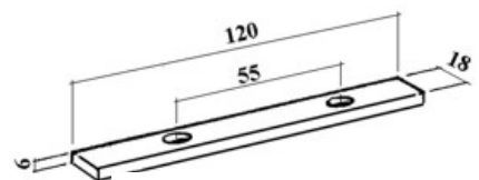
art. 15306 PIASTRINA gr. 100
