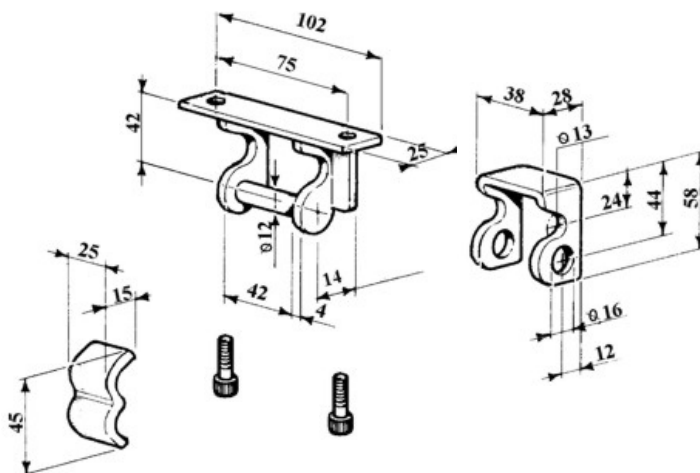
art. 15380 PALETTA LEGGERA gr. 33
