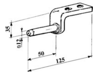
art. 15276 PERNO LEGGERO gr. 200
