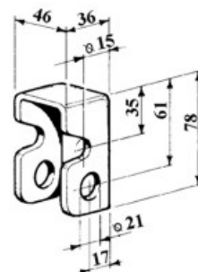
art. 15285 PIASTRINA gr. 95
