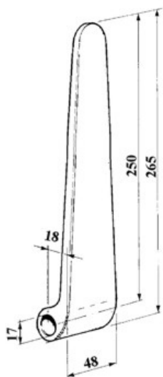
art. 15368 CERNIERA LAT. H265 gr. 740
