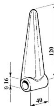
art. 15122 CERNIERA BOMBATA PESANTE gr. 250
