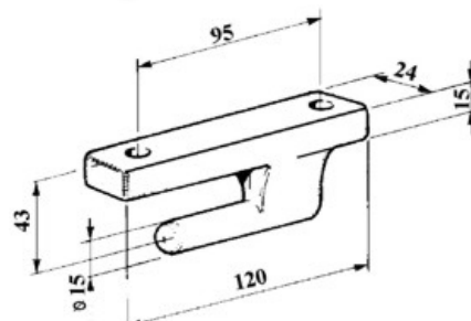
art. 15290 PERNO TIR PESANTE gr. 400
