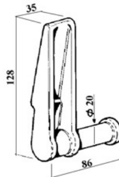
art. 15112 CERNIERA POST. PESANTE gr. 550
