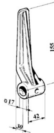
art. 15164 CERNIERA LAZIO gr. 640
