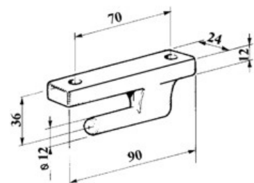
art. 15280 PERNO TIR LEGGERO gr. 230
