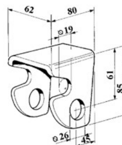
art. 15240 SUPPORTO GUIDA ASTA gr. 600
