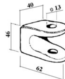
art. 15116 SUPPORTO PESANTE gr. 380
