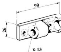
art. 15282 CERNIERA TIR LEGGERA gr. 190
