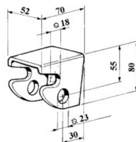
art. 15220 SUPPORTO GUIDA ASTA gr. 500
