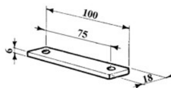
art. 15382 PIASTRINA gr. 80
