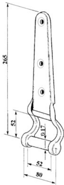
art. 15360 CERNIERA S/FORI GREZZA H265 gr. 770
