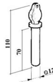
art. 15104 SPINOTTO D.12 gr. 110
