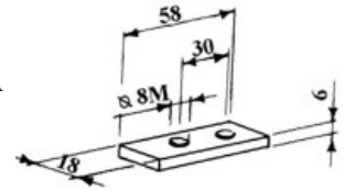
art. 15270 PIASTRINA gr. 40
