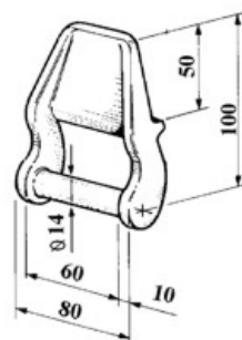
art. 15208 CERNIERA LEGGERA gr. 500
