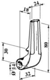
art. 15148 CERNIERA CORTA IN FUORI gr. 180
