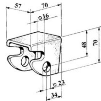
art. 15212 SUPPORTO gr. 430
