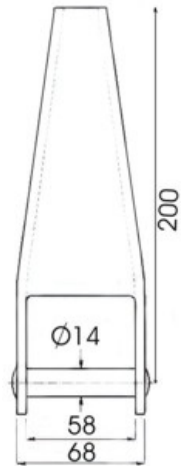
art. 15204 CERNIERA T/PARIPIANALE ALTA gr. 690
