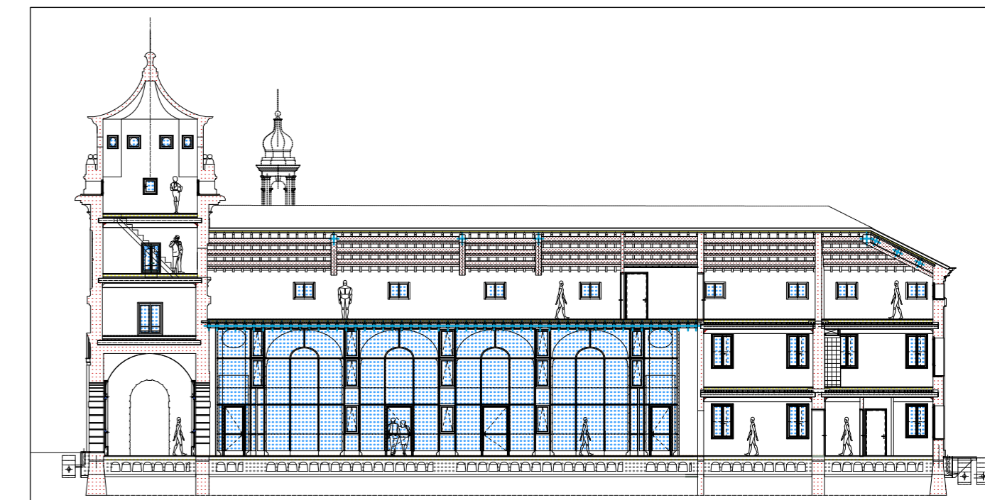
sezione h.h
