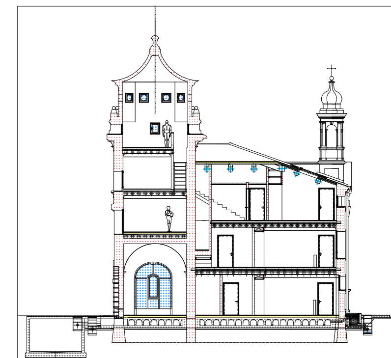
sezione d.d
