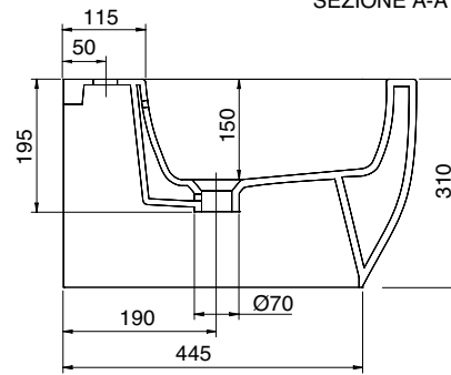
SEZIONE A-A
